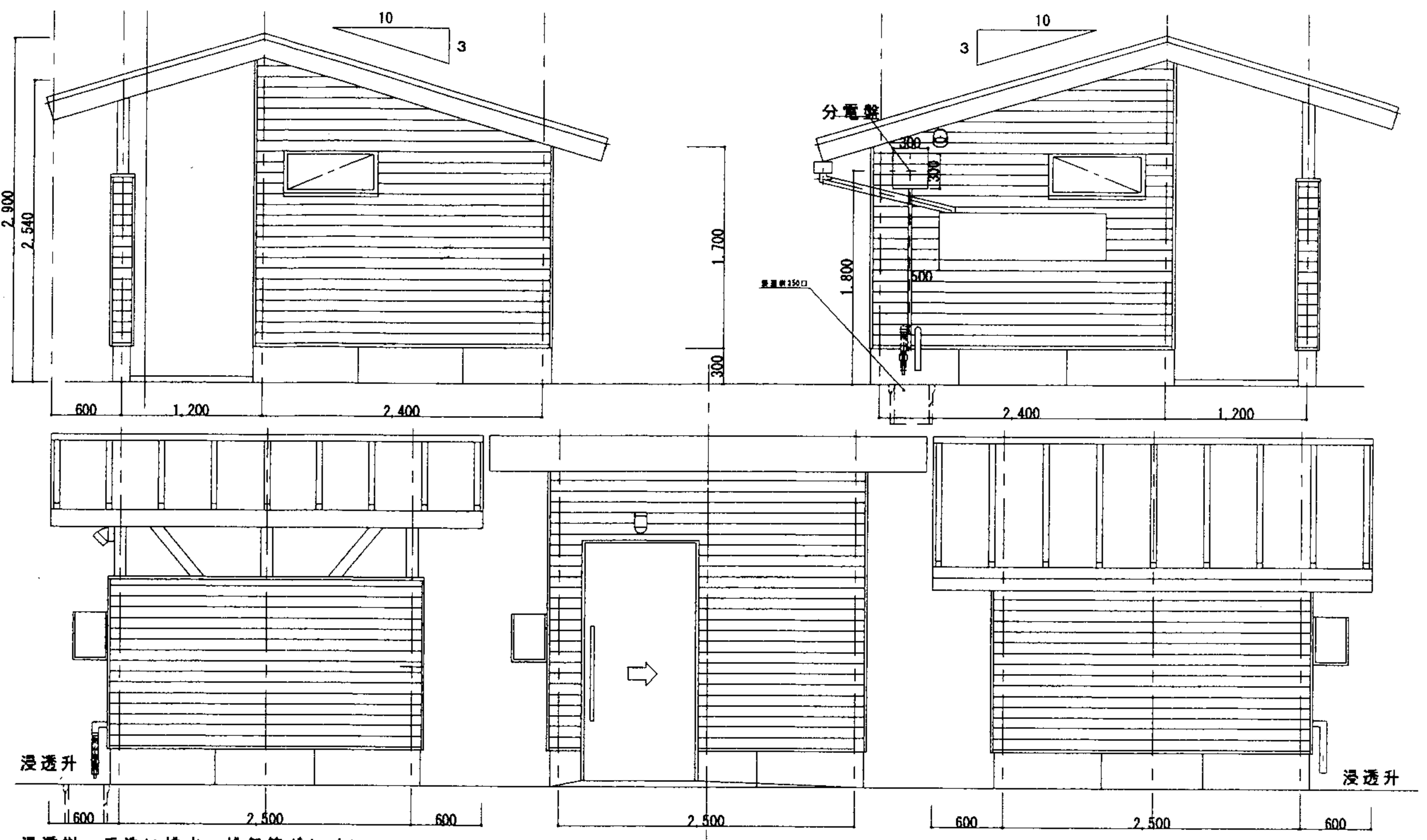
浸透柵、手洗い排水、排気筒ドレイン
