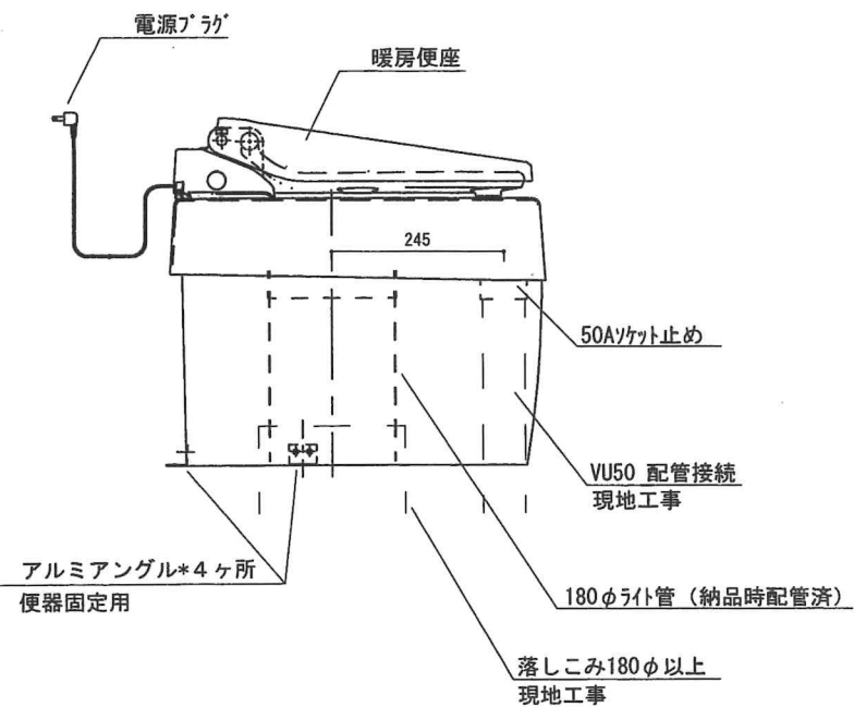
正面図
