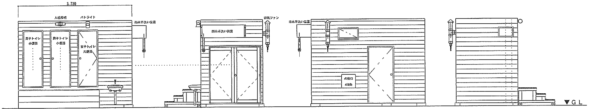
側面図 S=1/50
