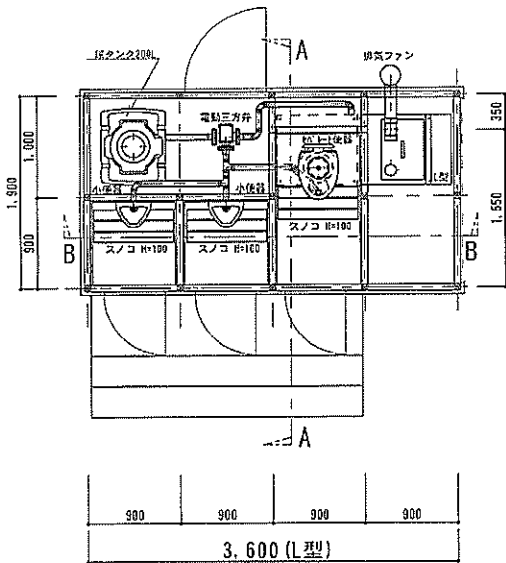
平面図 S=1/50
