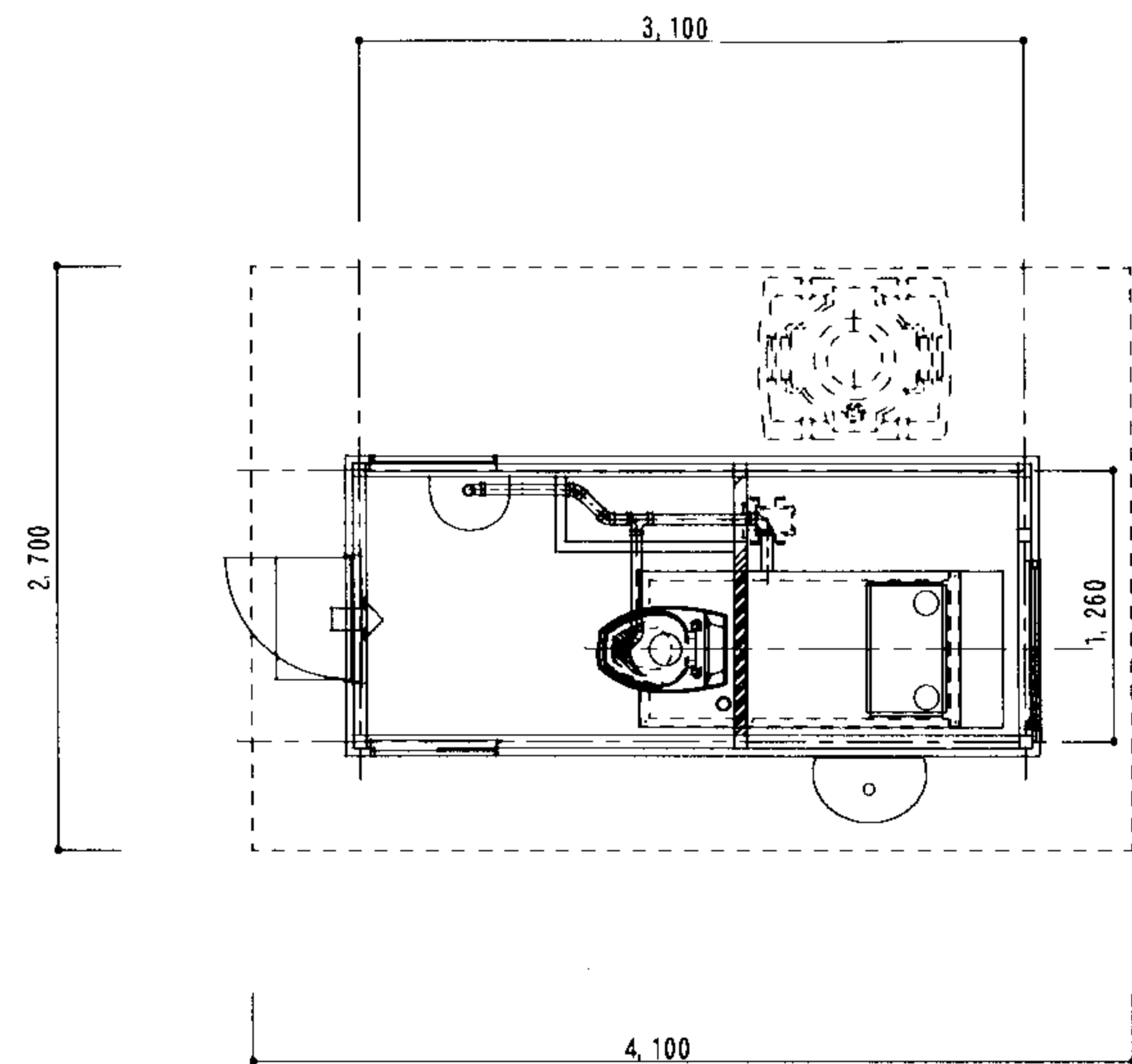
平面図 S = 1 / 5 0
