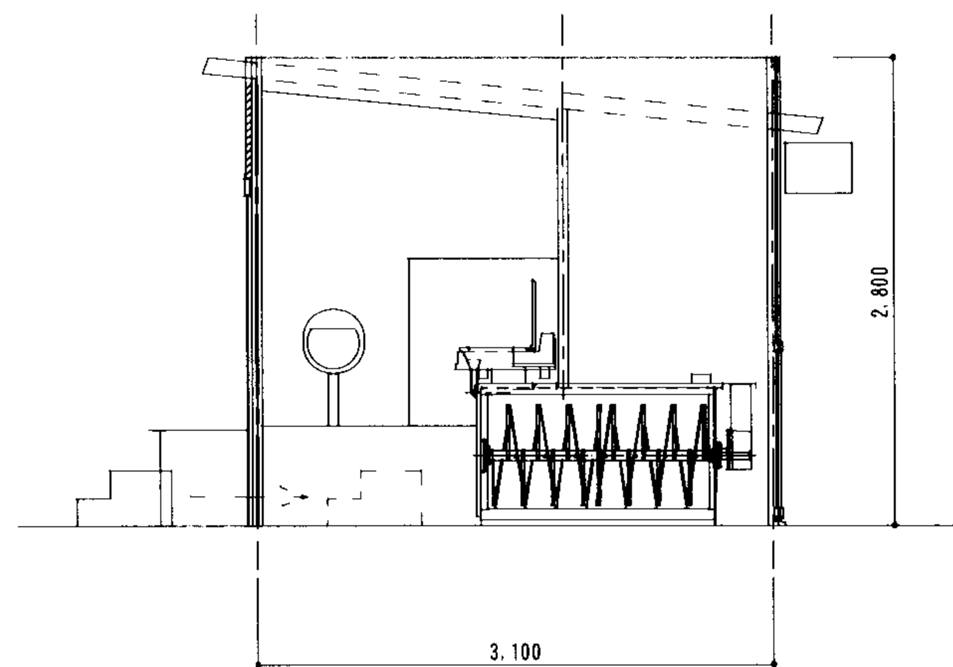
断面図 S = 1 / 5 0
