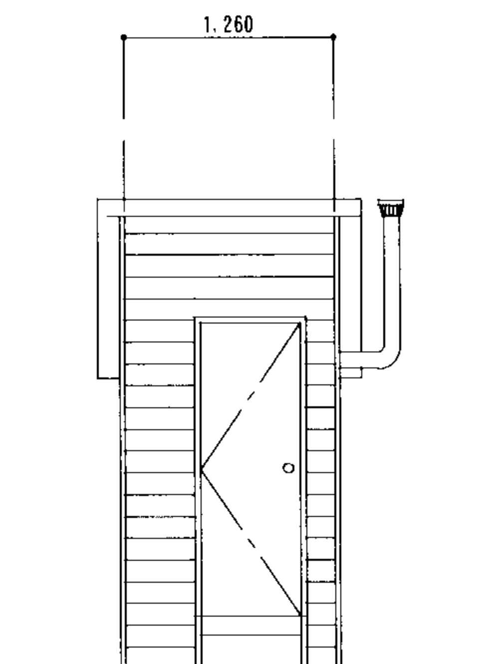
立面図 S = 1 / 5 0
