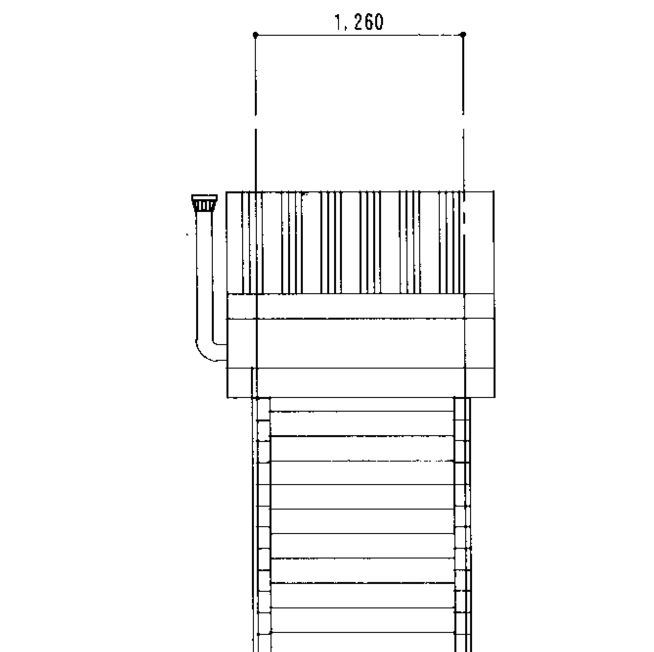
立面図 S = 1 / 5 0
